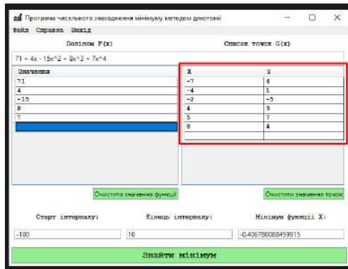
Рисунок 1 – Приклад обчислення мінімуму функції
